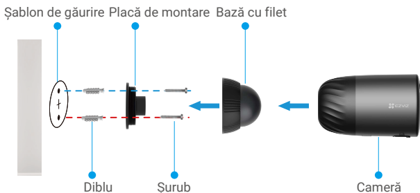
Fig. 2 Securizat cu baza magnetică
