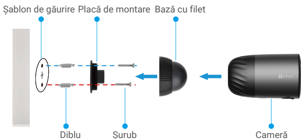
Fig. 1 Securizat prin bază cu șurub
